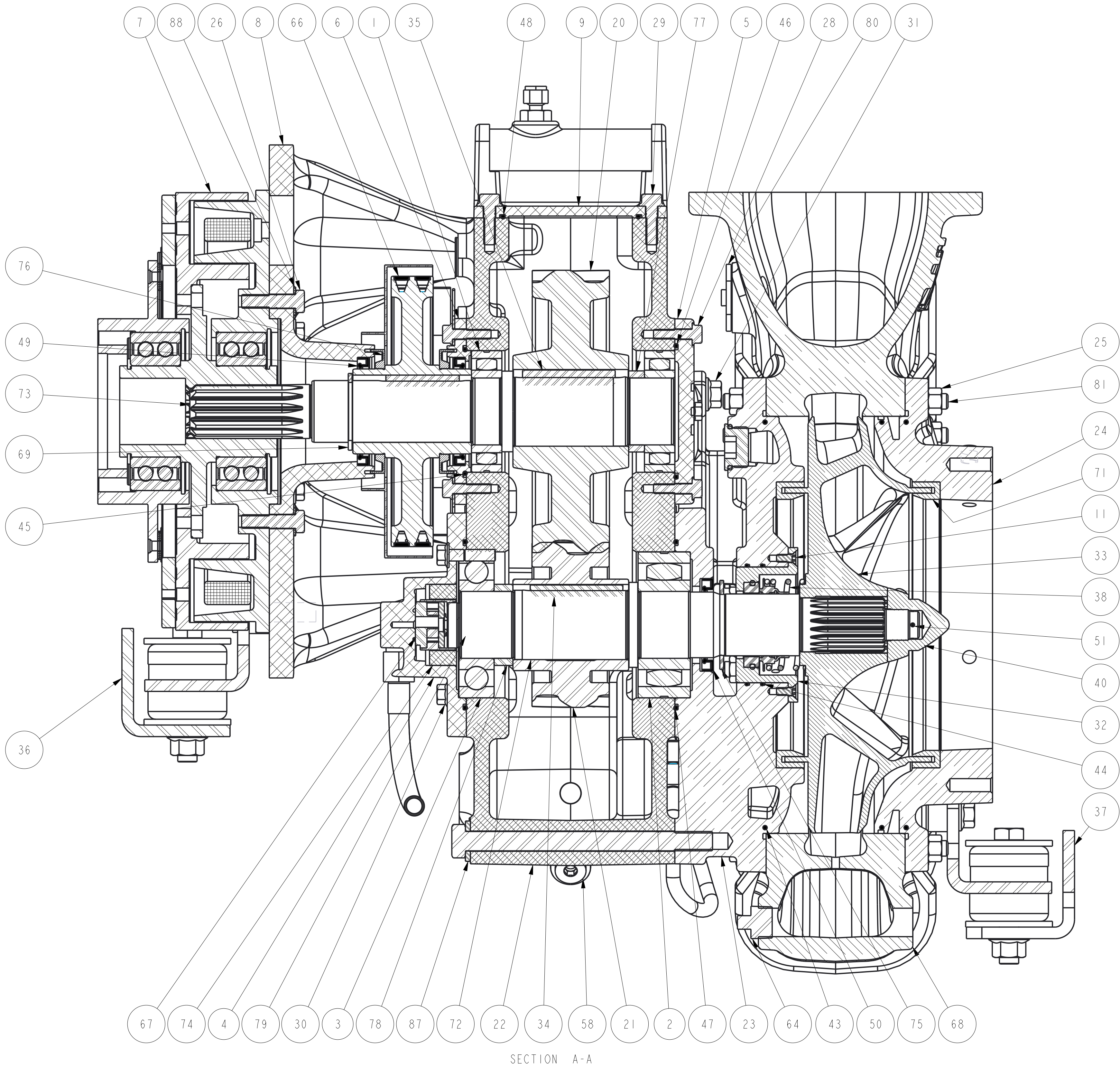
SECTION A-A
