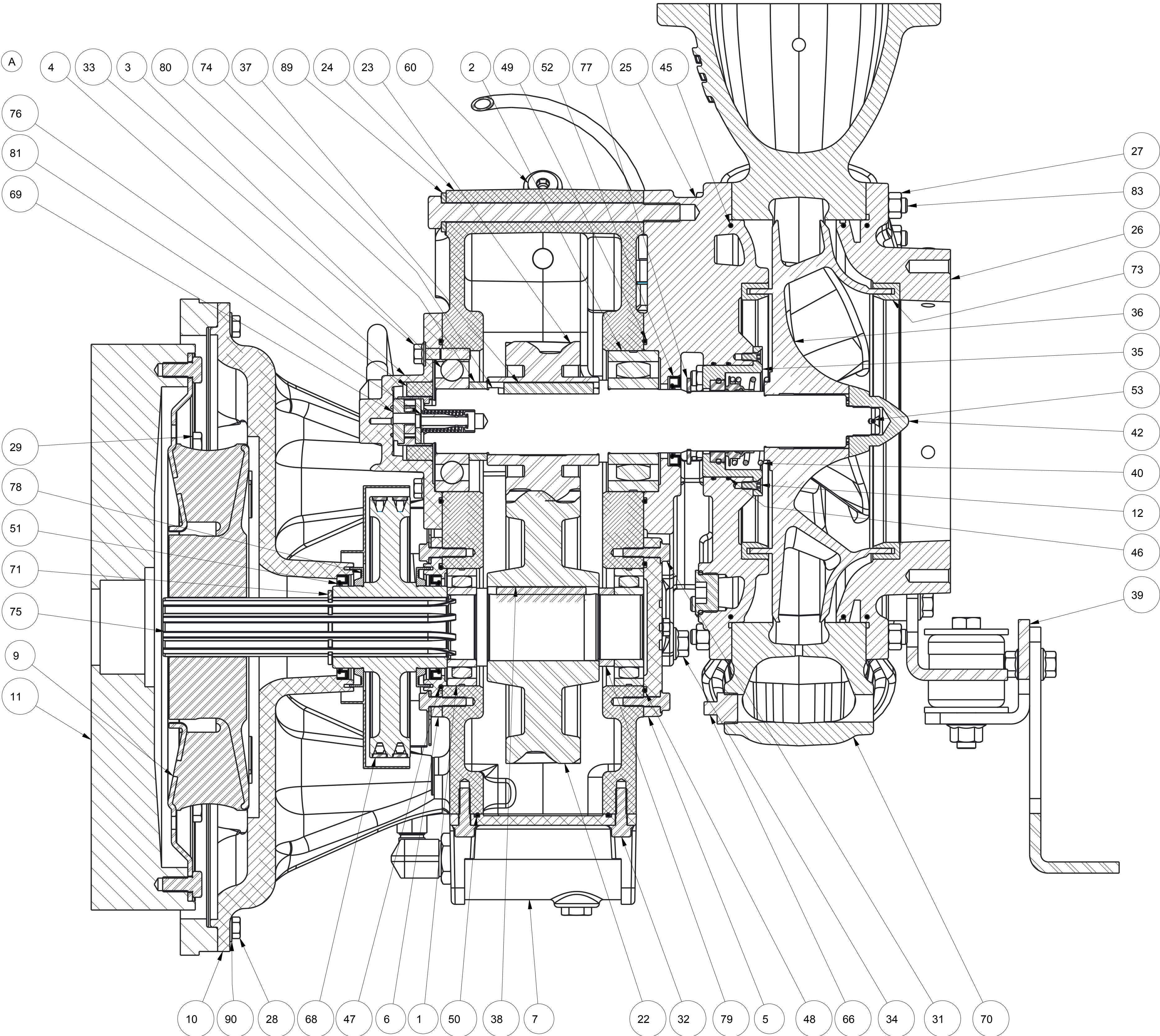
SECTION A-A
