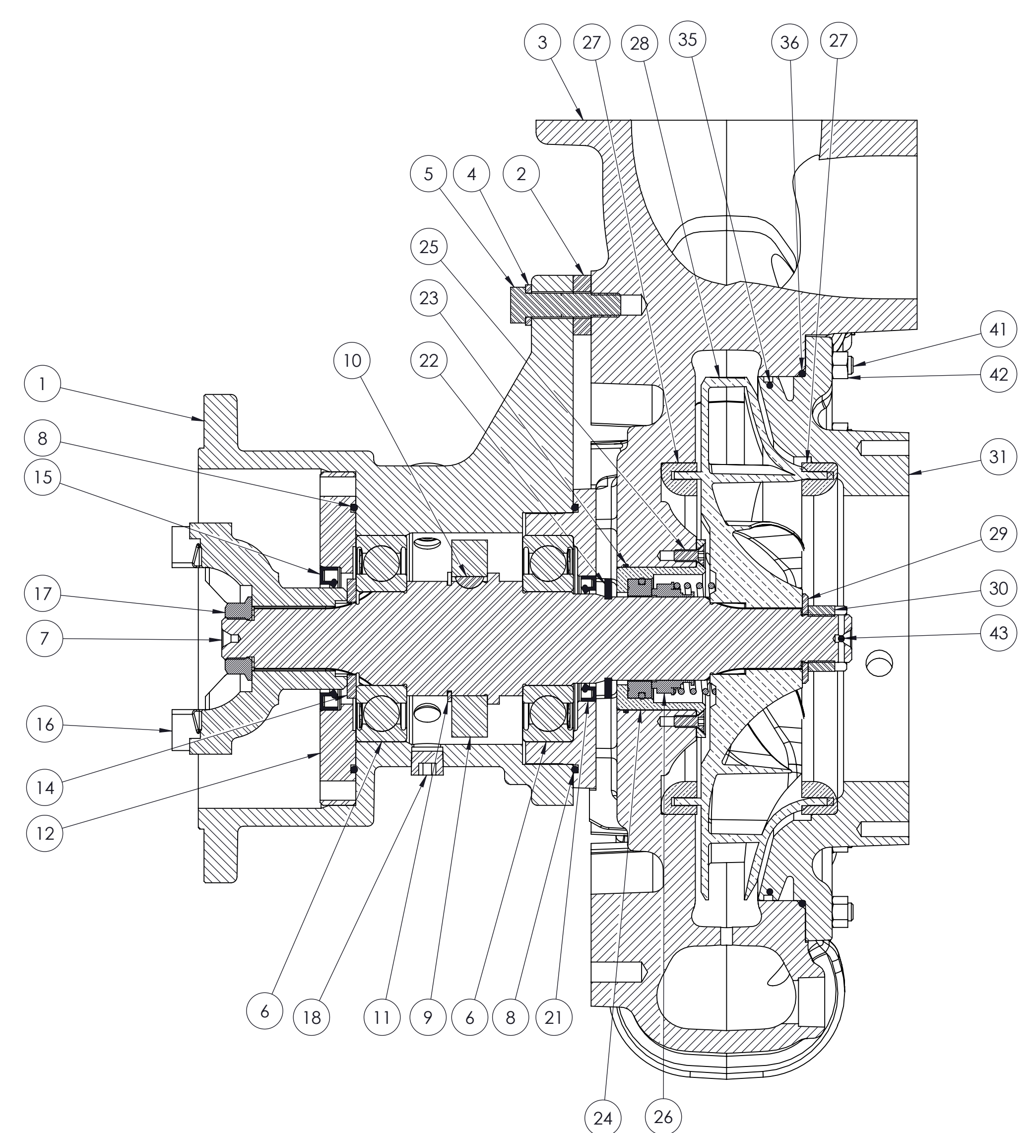
SECTION A-A
