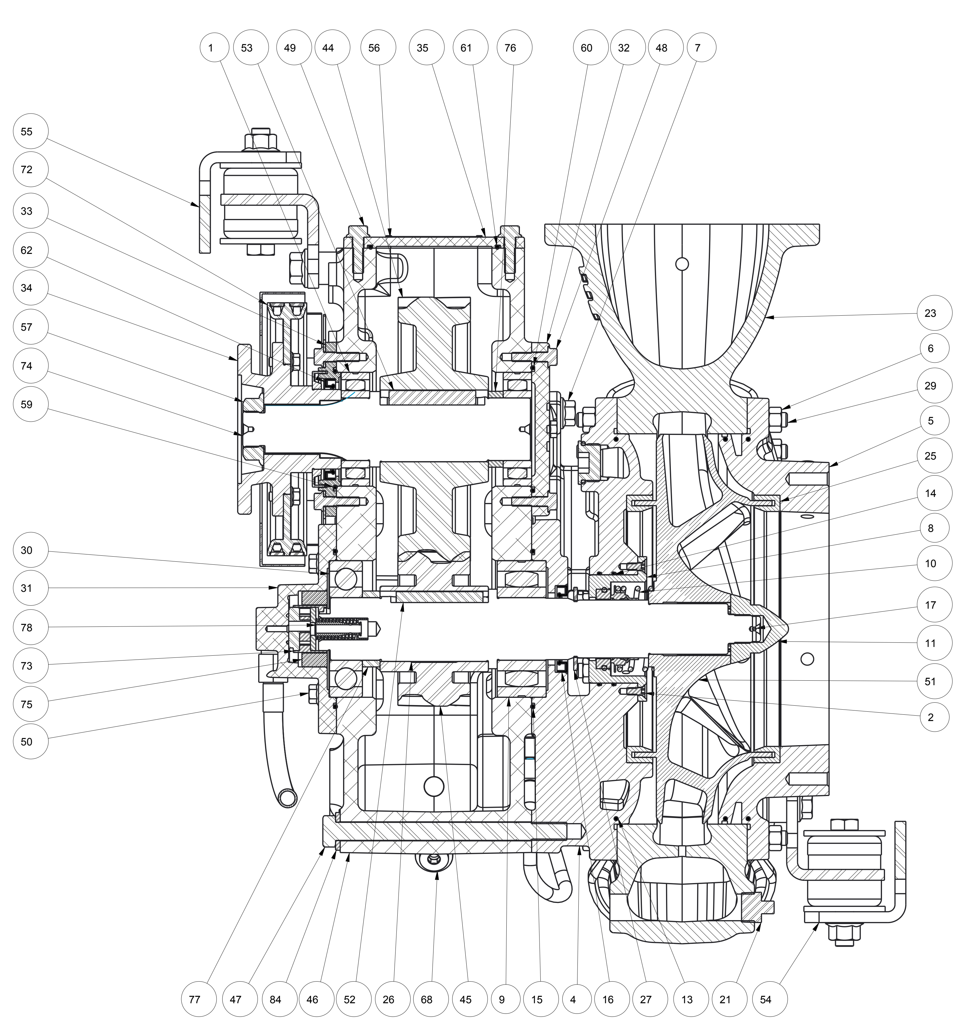
SECTION A-A
