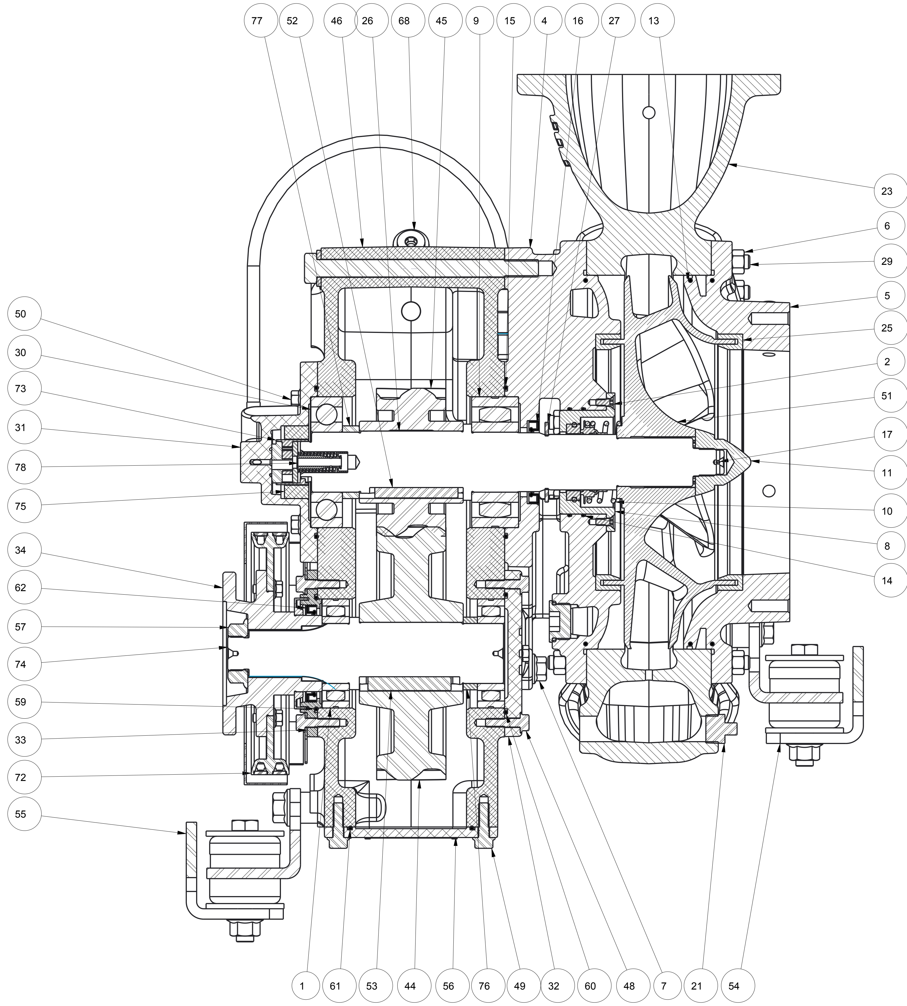
SECTION A-A
