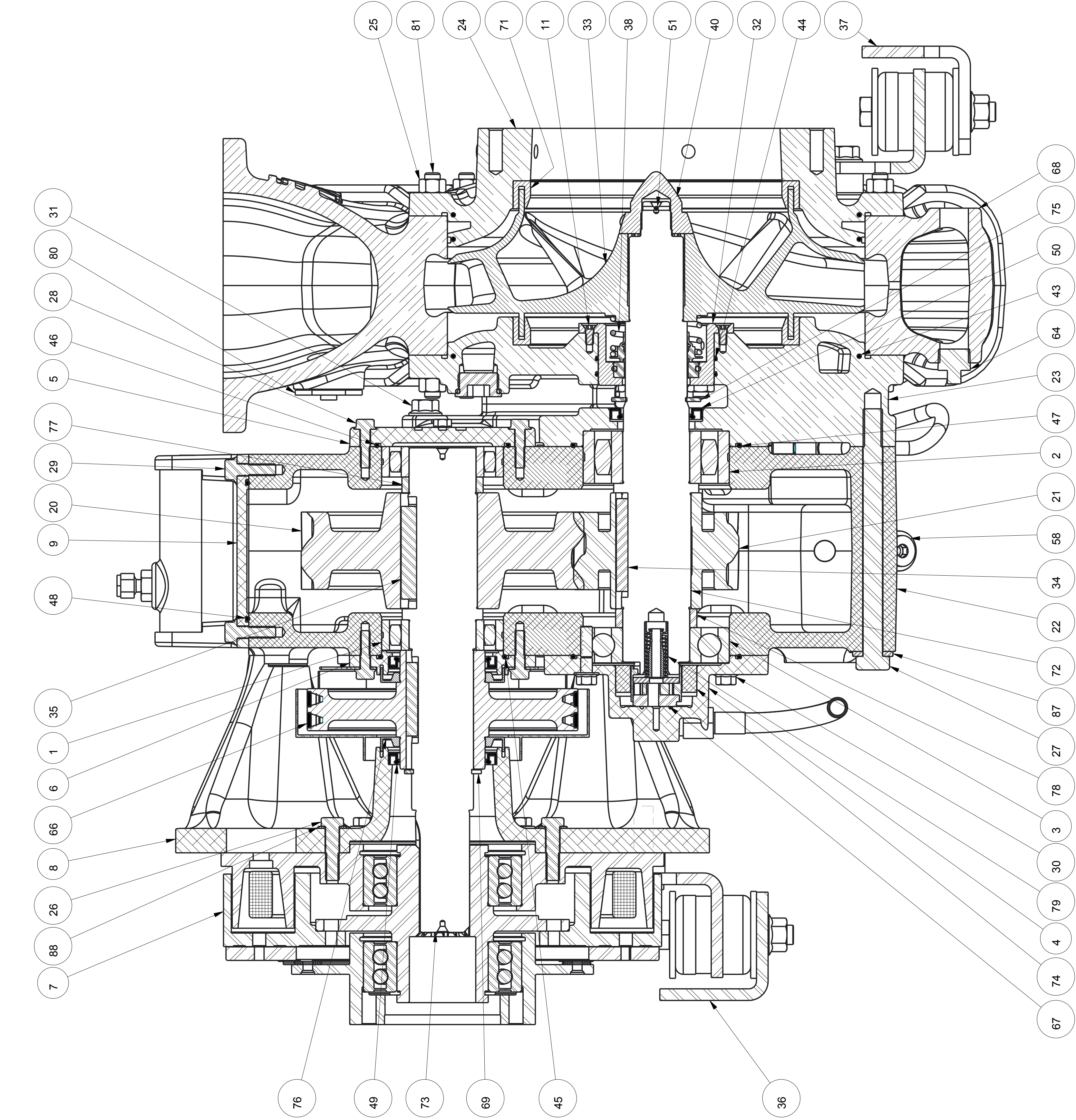
SECTION A-A
